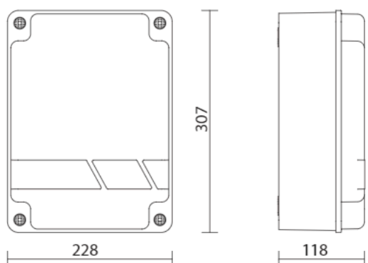
Dimensions R70/2AC/BOX
