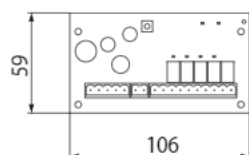
Dimensions H85/DEC/BOX
